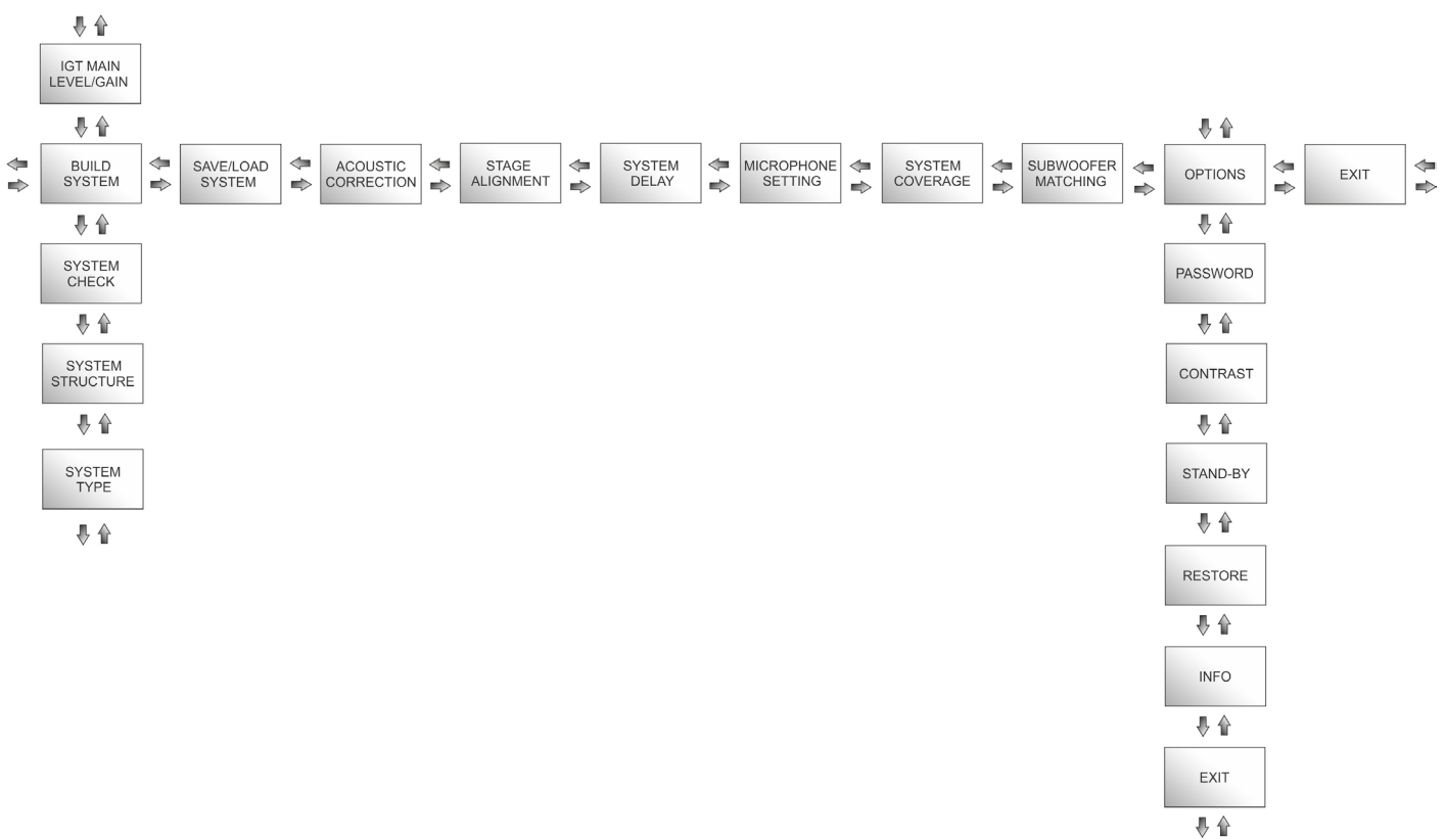
Menu
